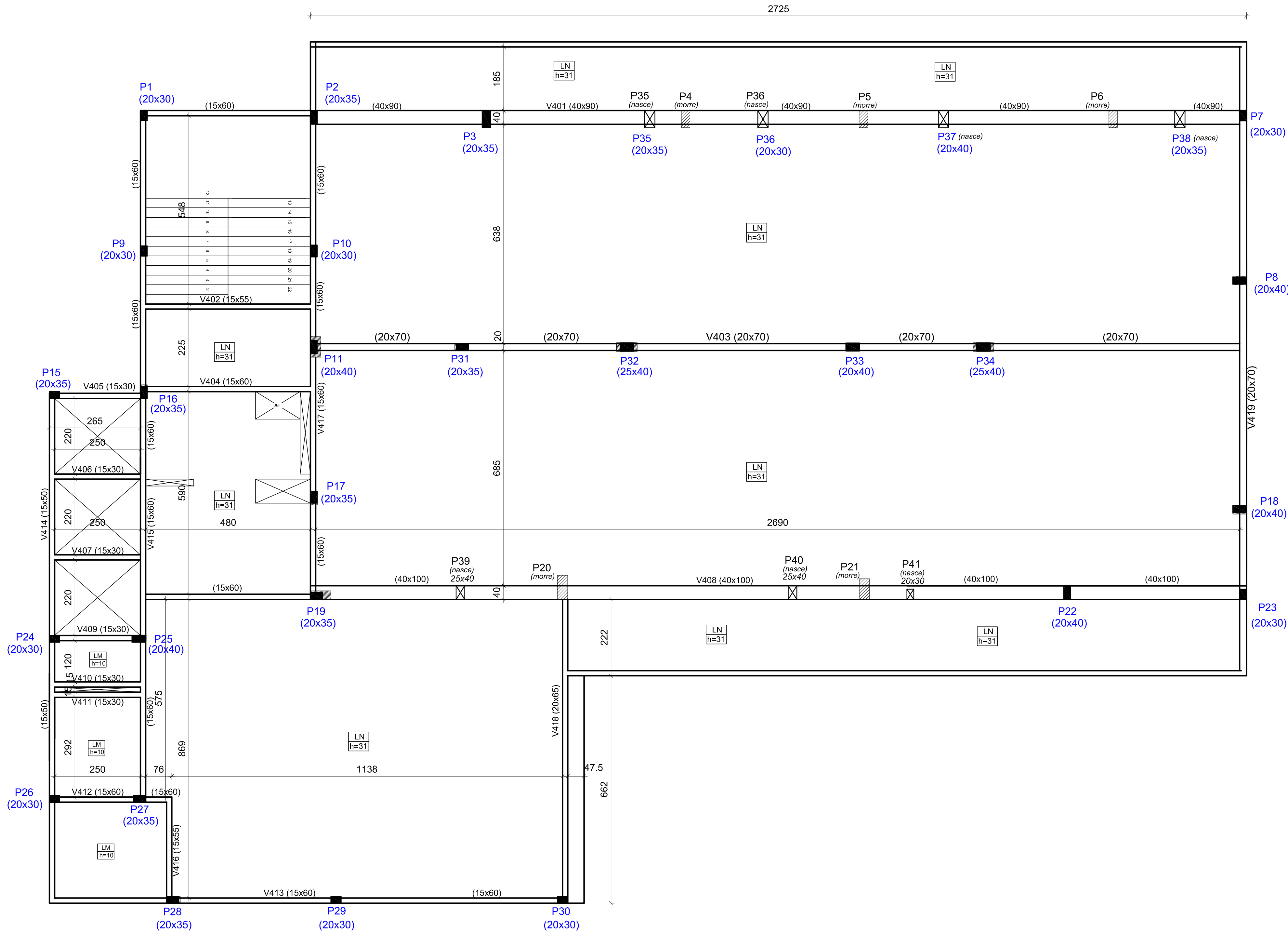
Planta de Fôrmas - 5º Pavimento Escala 1:50
